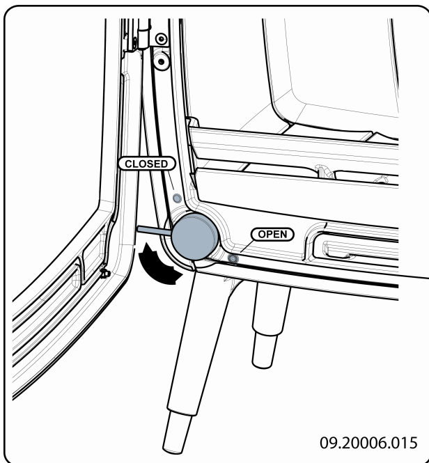
Primaire luchtschuif
