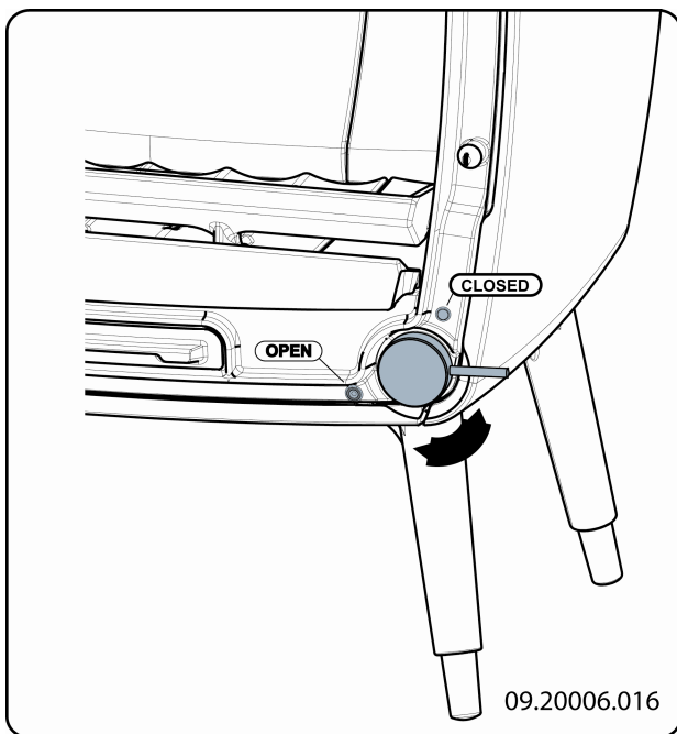
Secundaire luchtschuif
